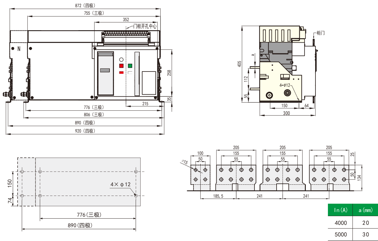
12、RIVW1-6300、6300/4 In=4000、5000抽屉式断路器安装尺寸及外形尺寸
