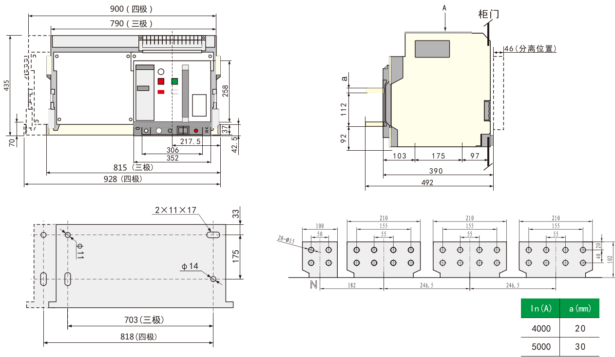
12、RIVW1-6300、6300/4 In=4000、5000抽屉式断路器安装尺寸及外形尺寸
