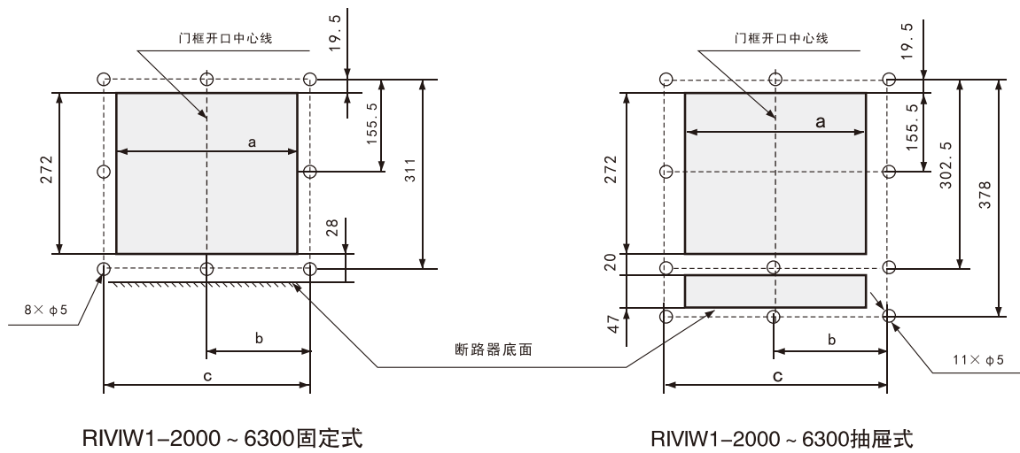
16、面板开孔安装尺寸图
