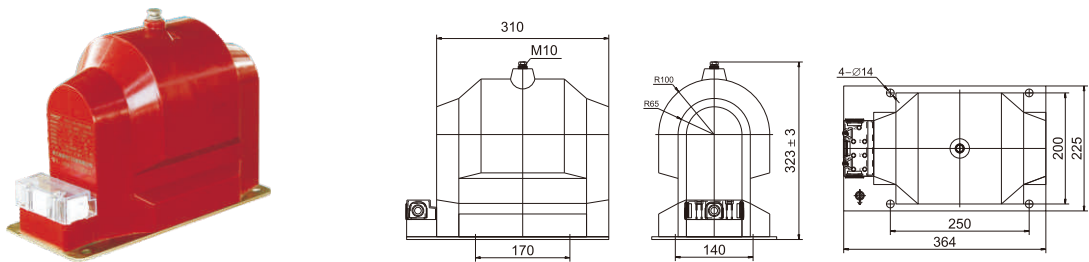
JDZX9-20单相全封闭半绝缘浇注电压互感器
